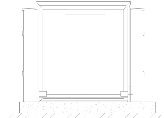
ELEVATION A
