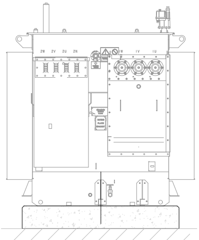
ELEVATION A
