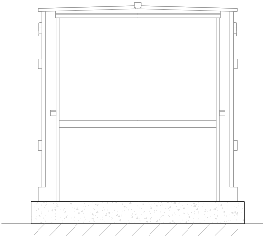
ELEVATION B
