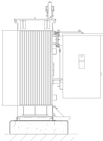
ELEVATION B
